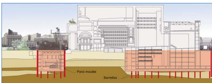
Coupe de l'ouvrage
